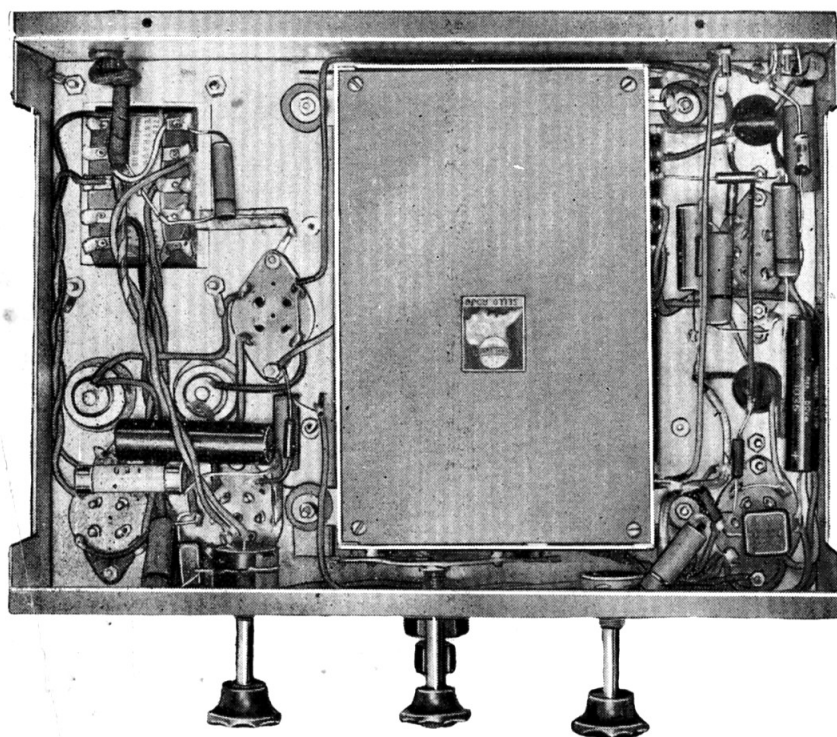
Chassis visto de abajo
